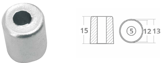
2626441 Anode
